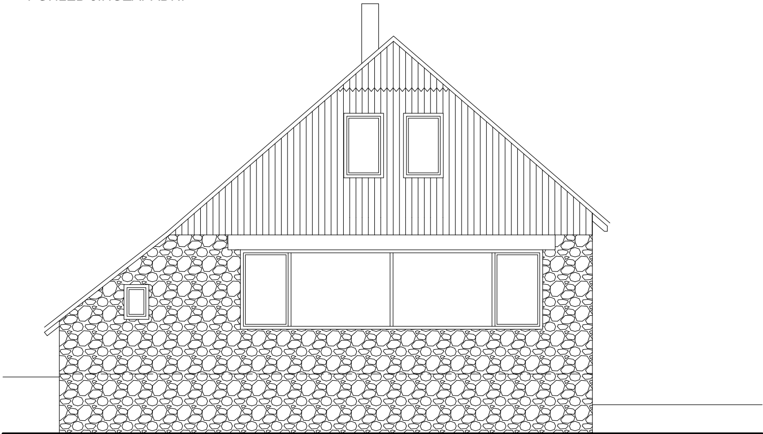
POHLED JIHOZÁPADNÍ
